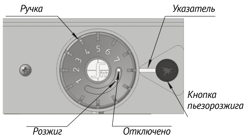
Рисунок 3. Устройство газогорелочное с газовым блоком 630 EUROSIT и TGV-307
