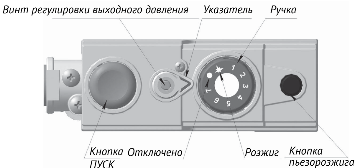
Рисунок 6. Элементы управления на газовом блоке автоматики САБК-АТ
