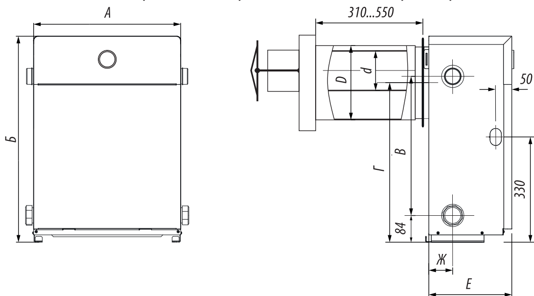
Рисунок 1. Общий вид, габаритные и присоединительные размеры котлов
